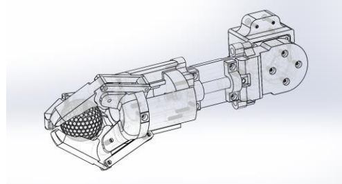
Fig. 3. Gripper
